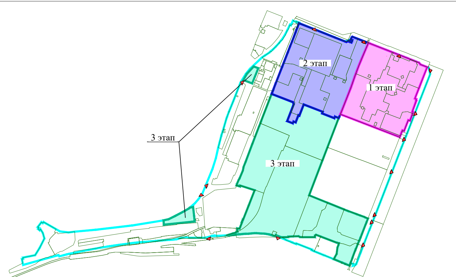
СХЕМА ЭТАПОВ РАЗРАБОТКИ ПРОЕКТА МЕЖЕВАНИЯ ТЕРРИТОРИИ
