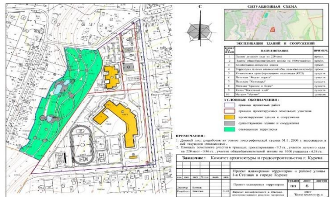
Проект планировки в районе ул. 1-я Степная
